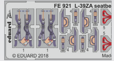
FE921 L-39ZA seatbelts STEEL 1/48 Trumpeter (1 část)
