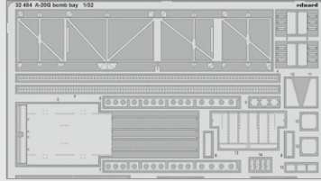
32484 A-20G bomb bay 1/32 HKM (1 část)
