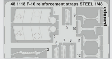
481118 F-16 reinforcement straps STEEL 1/48 Kinetic (1 část)
