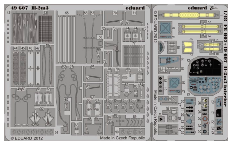
49607 II-2m3 S.A.
